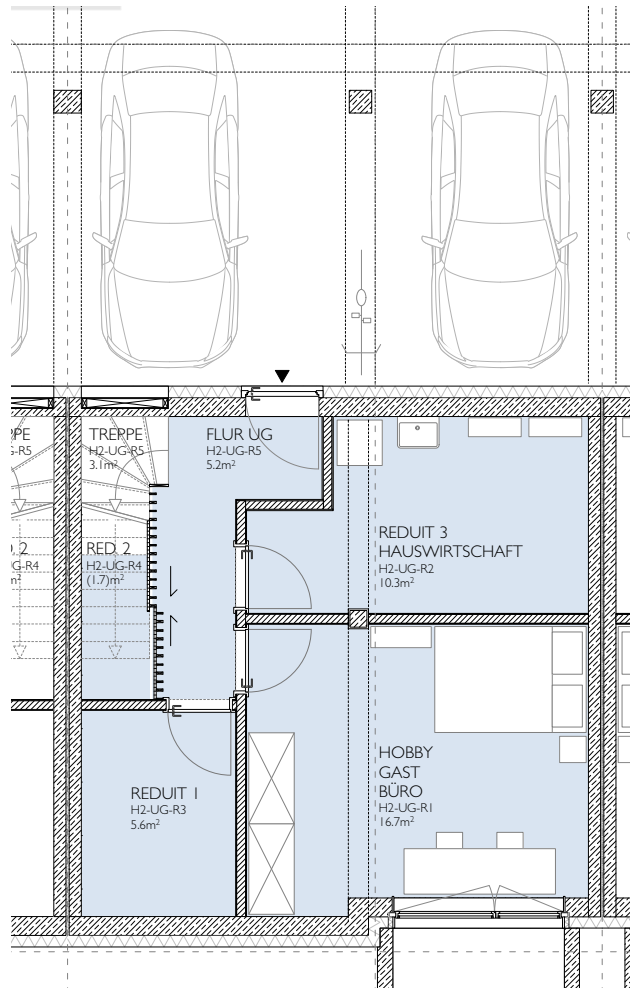
Untergeschoss
